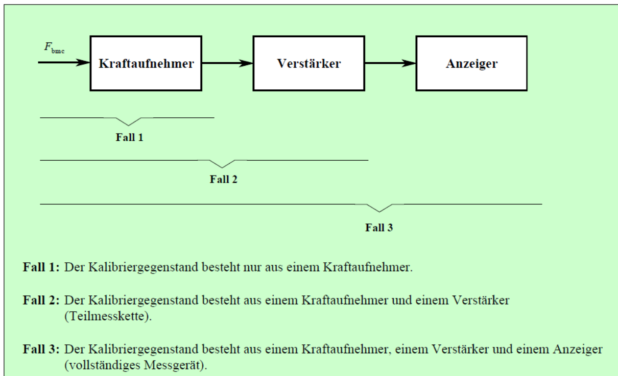
Fallunterscheidung Kalibriergegenstand
