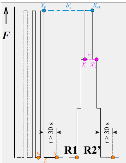
Kalibrierablauf C
