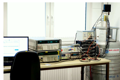
AC/DC-Josephson-Quantenvoltmeter
