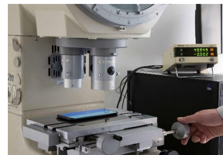
Das Smartphone wird horizontal unter dem Koordinatenmessgerät ausgerichtet.
